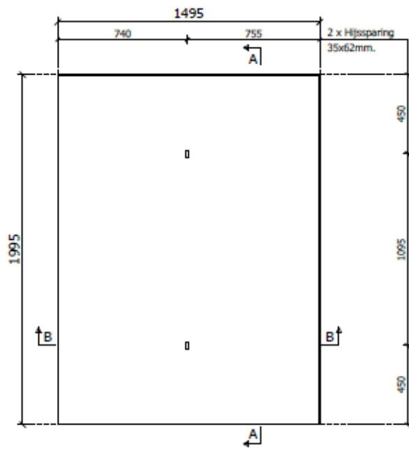
Bovenaanzicht (malzijde)
