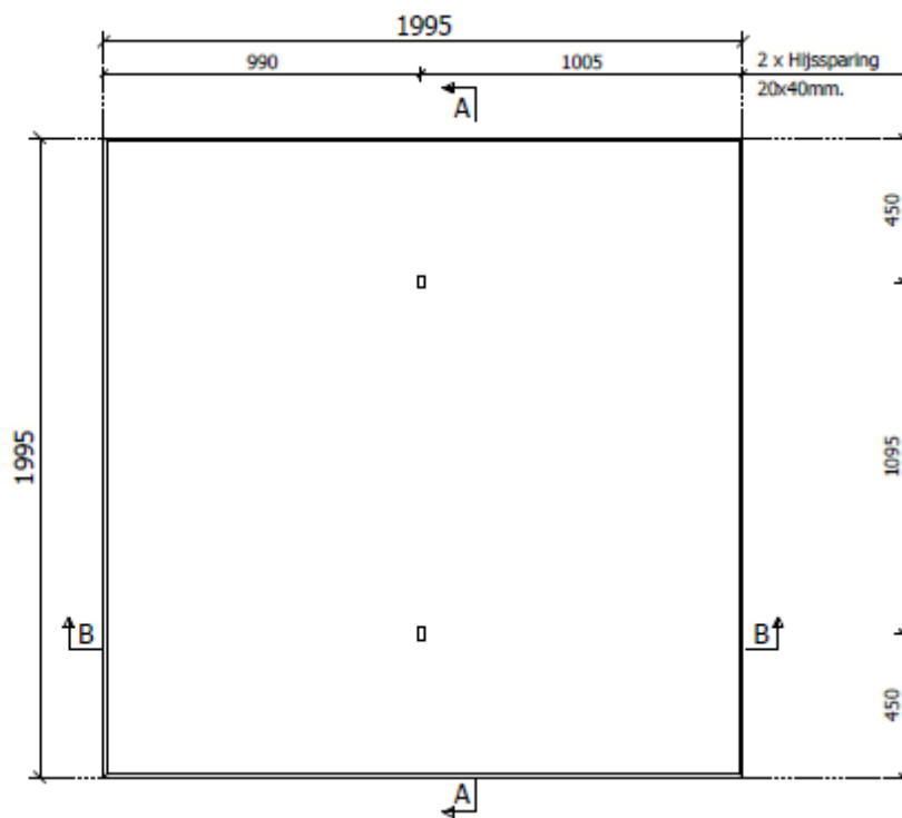
Bovenaanzicht (malzijde)
