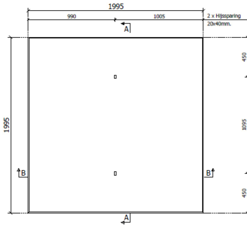
Bovenaanzicht (malzijde)
