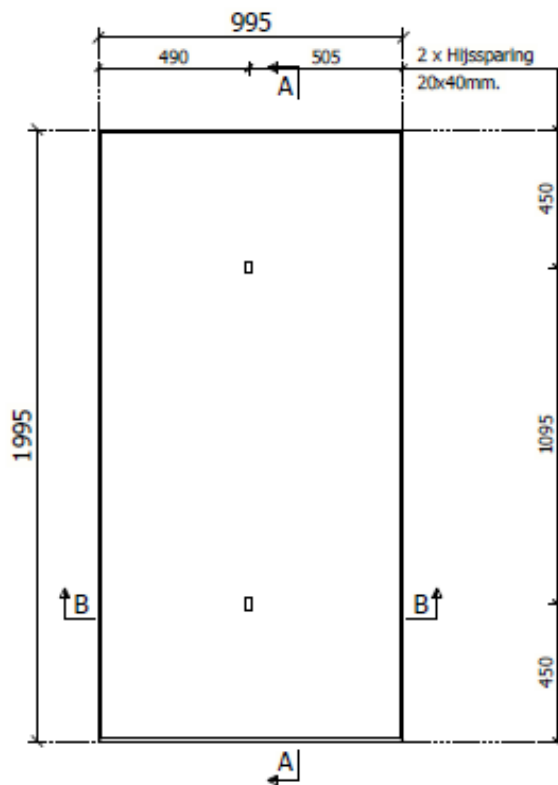
Bovenaanzicht (malzijde)
