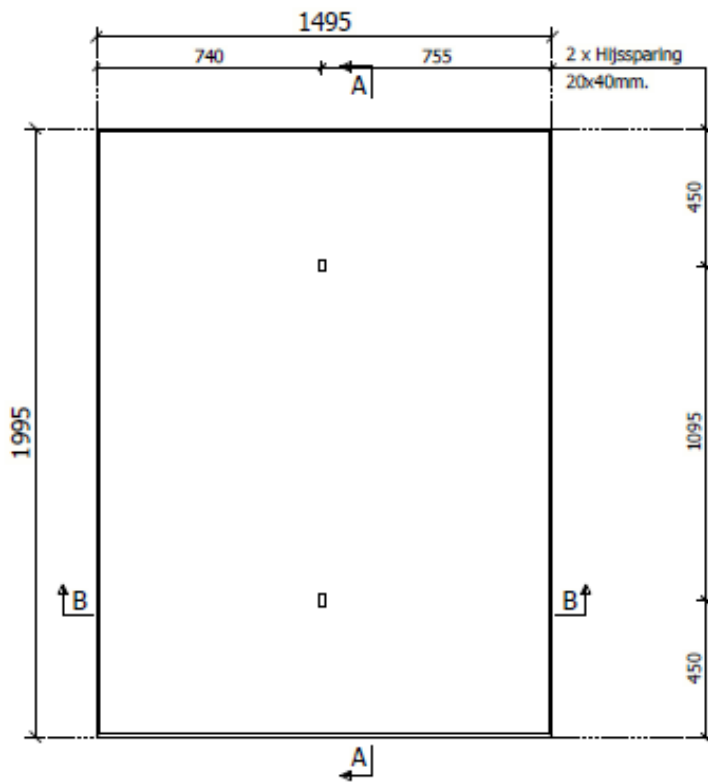
Bovenaanzicht (malzijde)
