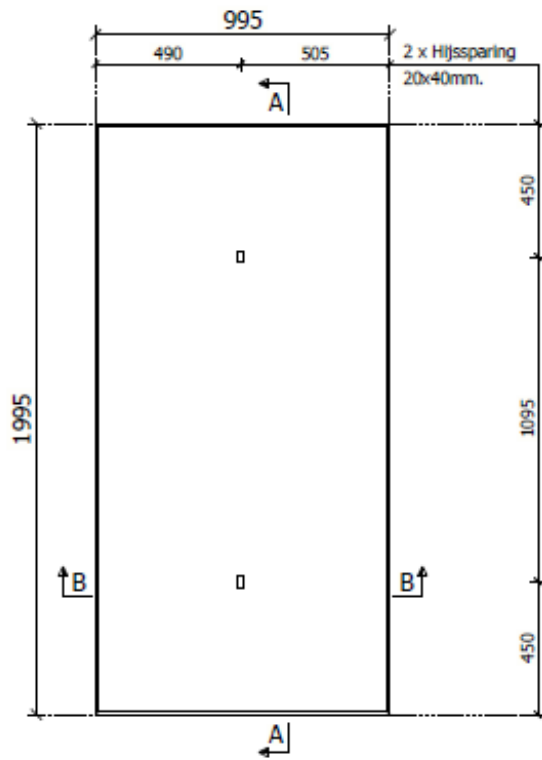
Bovenaanzicht (malzijde)
