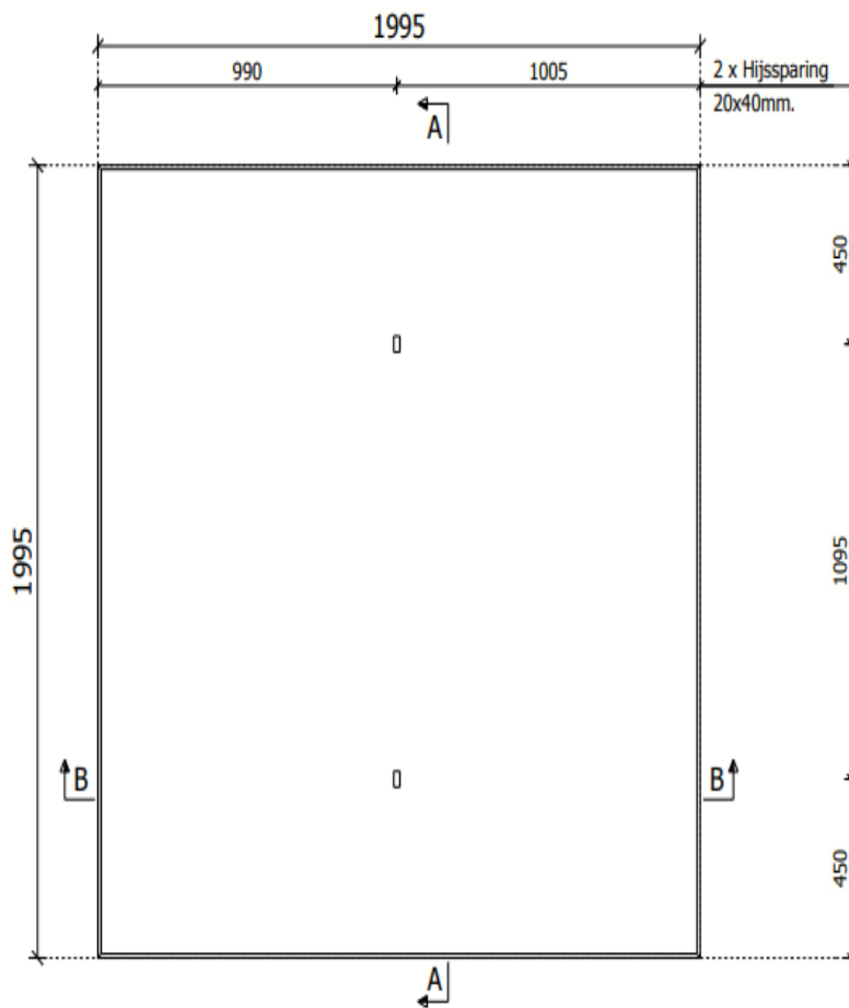
Bovenaanzicht (malzijde)
