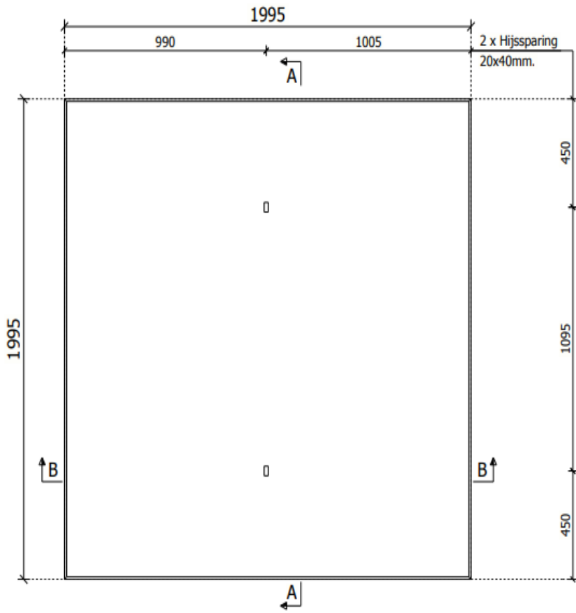
Bovenaanzicht (malzijde)
