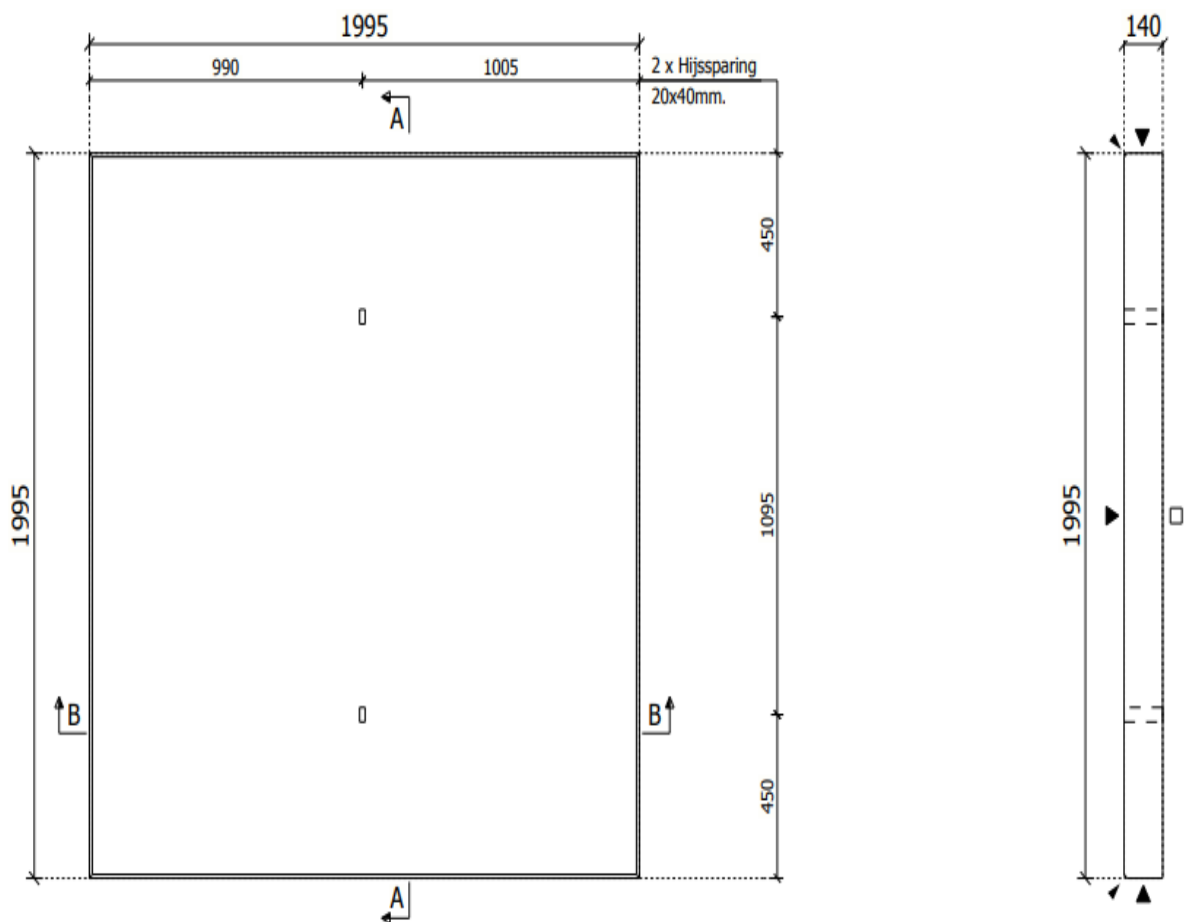
Bovenaanzicht (malzijde)
