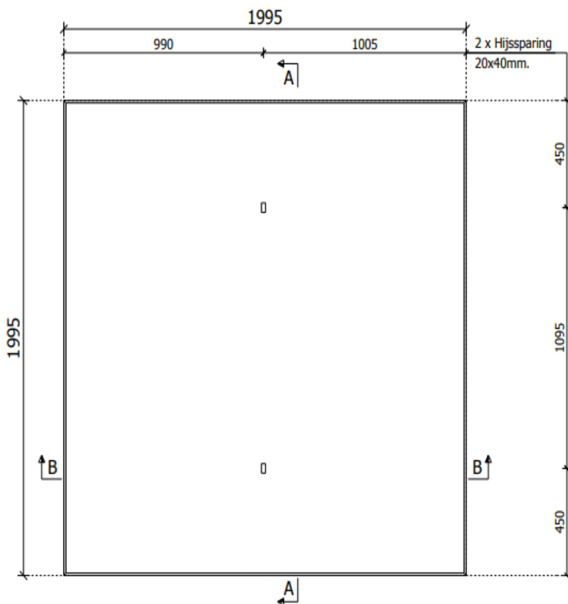
Bovenaanzicht (malzijde)
