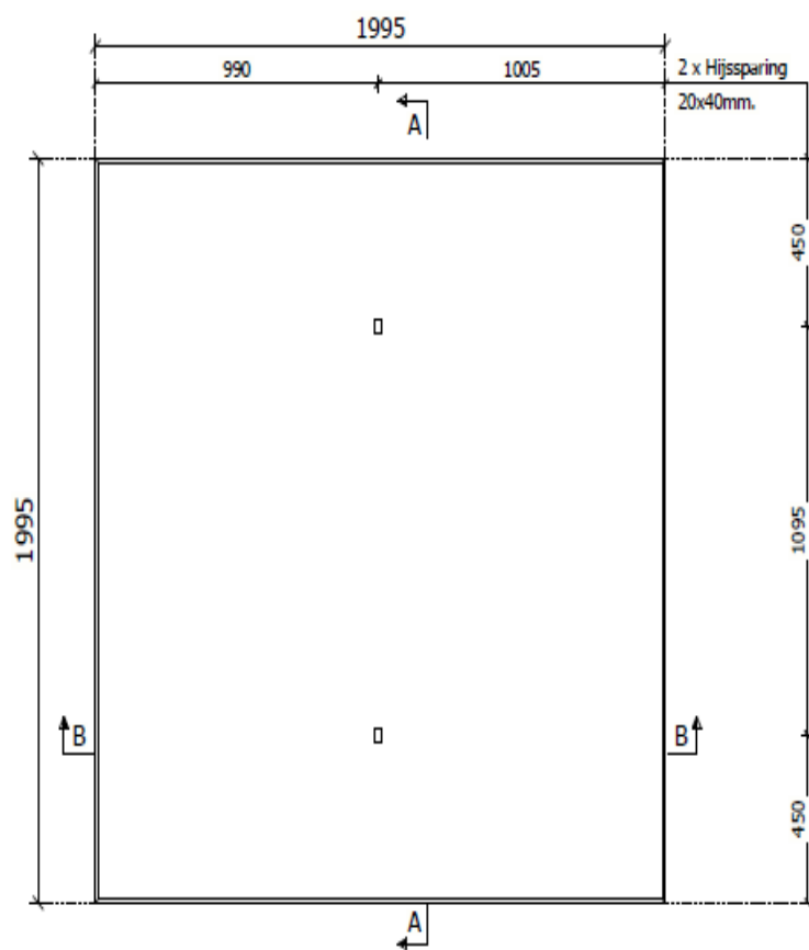
Bovenaanzicht (stortzijde)
