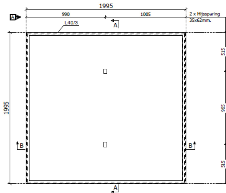
Bovenaanzicht (stortzijde)
